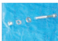
VIS M8x40 TCEI ZN RONDELLE 8,4x16 H1,6 ZN ÉCROU DE SÉC. M8 ZN
